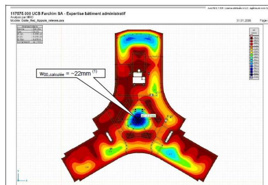
Modèle numérique des déformations calculées
