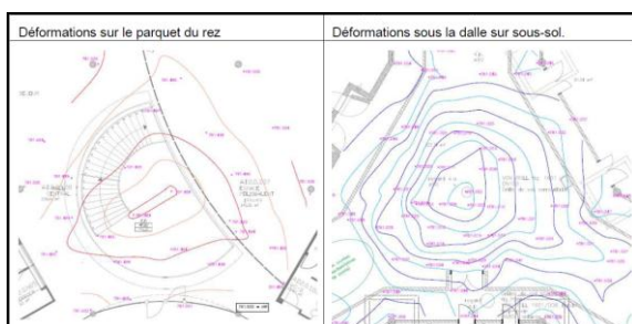
Modèle numérique des déformations mesurées
